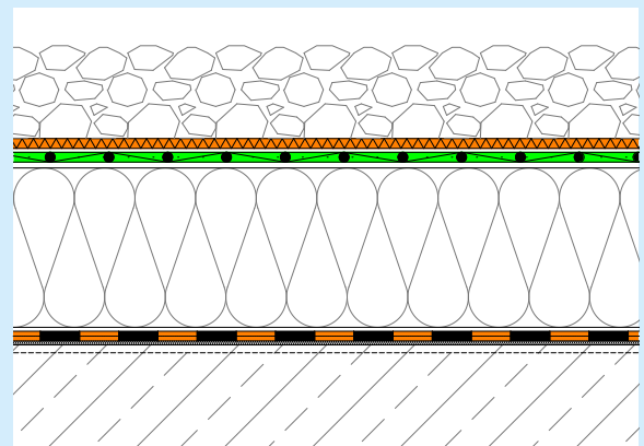
Lose verlegt unter Auflast
