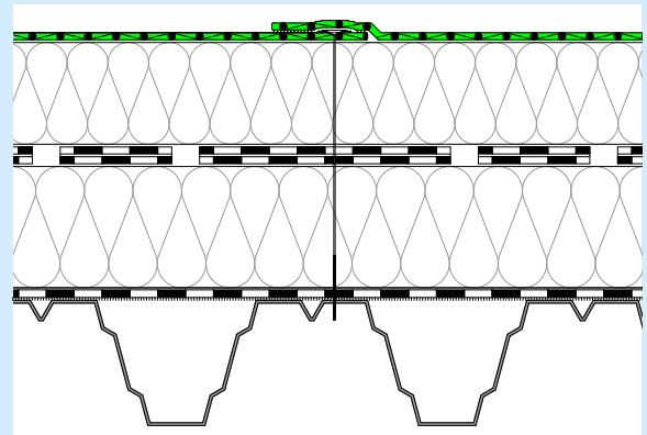
Mechanisch befestigter Schichtenaufbau, auch bei der Sanierung feuchter Altdachschichten
