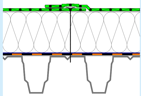
Mechanisch befestigter Schichtenaufbau
