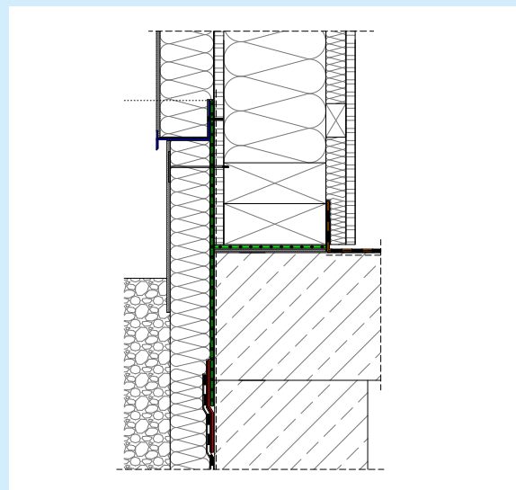
Spritzwasserschutz im Sockelbereich
