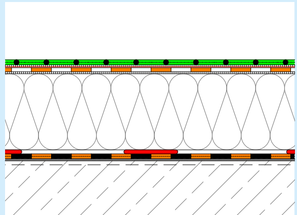
Geklebter Schichtenaufbau
