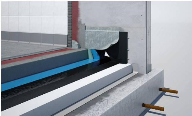
Innenraumabdichtung Küche
