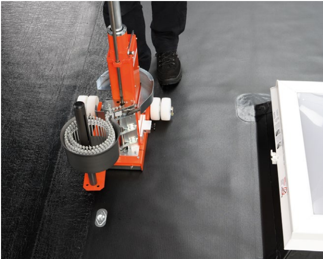
Rationelle Befestigung der Drill-Tec Flachdachbefestiger mit einem professionellen Setzautomaten
