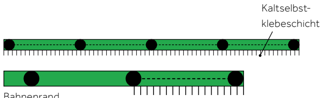
Bahnenrand Bahnen­aufbau Wolfin GWSK
