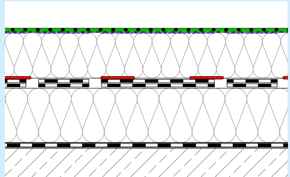
Geklebter Schichtenaufbau mit perforierter Altabdichtung
