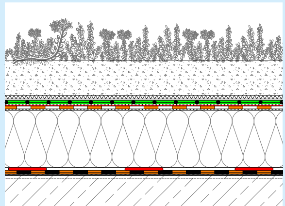
Geklebter Schichtenaufbau unter Auflast
