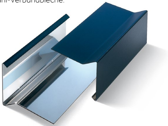
Verbundbleche für linienförmige Befestigungen
