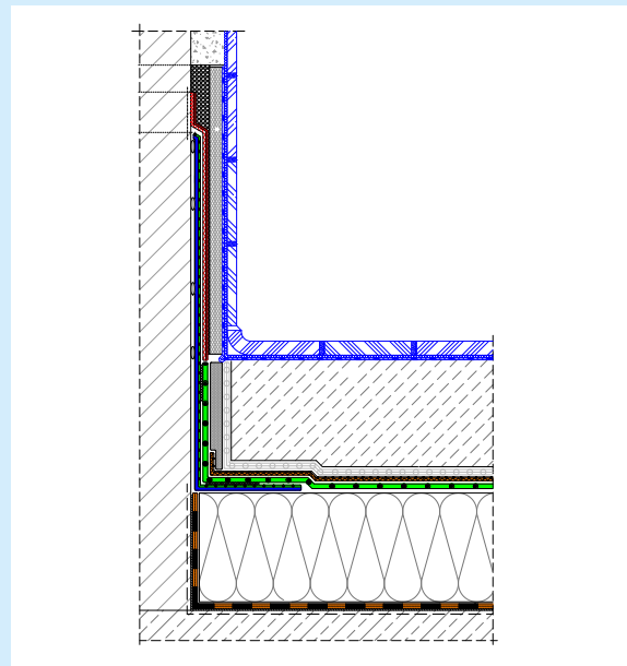
Bauwerksschutz unterhalb des Estrichs in der Küche
